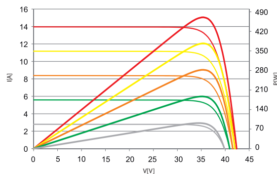
CHARAKTERYSTYKA PRĄDOWO-NAPIĘCIOWA
